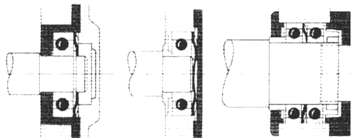
Einbaubeispiele: Kugellagerausgleichsscheiben
